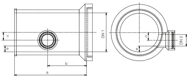
PROVEDENÍ: HLAVNÍ POTRUBÍ S HRDLEM/PŘÍTOK S HRDLEM
