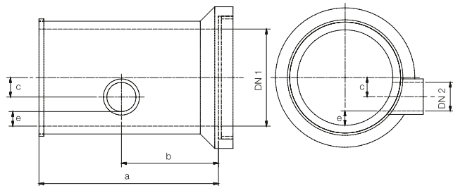
PROVEDENÍ: HLAVNÍ POTRUBÍ S HRDLEM/PŘÍTOK S HLADKÝMI KONCI
