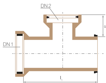
Ramificație 90°
