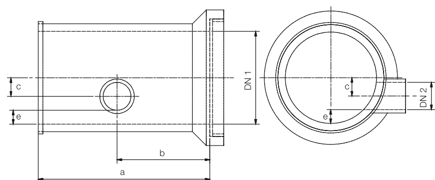
Ramificație excentrică: conductă principală cu mufă/admisie fără mufă
