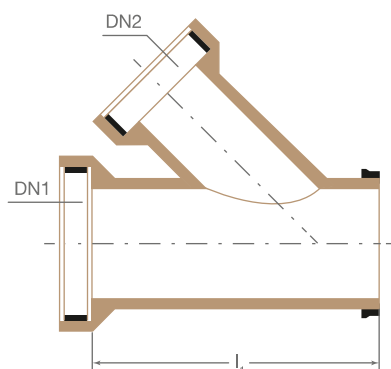
Ramificație specială 45° DN 1 cu mufă și DN 2 cu mufă
