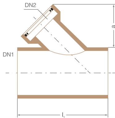
Ramificație reparație 45°
