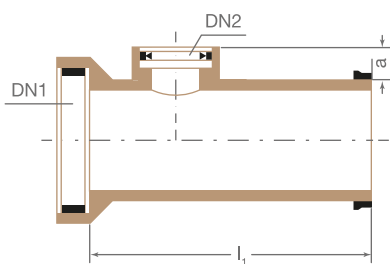
Ramificație compactă 90°
