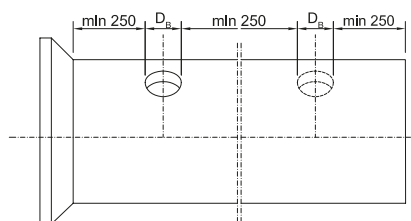
D_B = Diametru gaură de foraj
