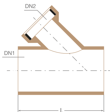
Ramificație specială 45° DN 1 fără mufă și DN 2 cu mufă
