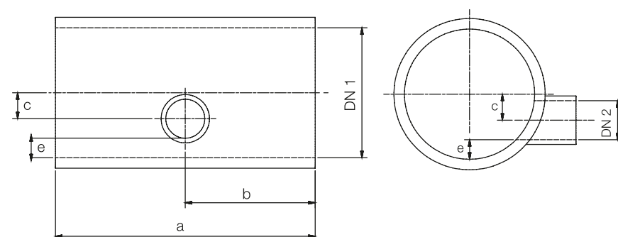
Ramificație excentrică: conductă principală fără mufă/admisie fără mufă
