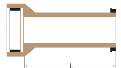
Piesă articulată admisie (GZ)
