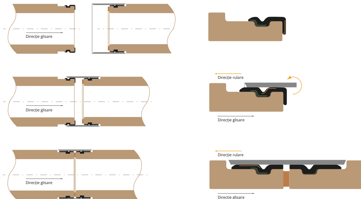
Principiul de funcționare a garniturii inelare cu alunecare
