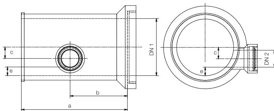
Ramificație excentrică:: conductă principală cu mufă/admisie cu mufă
