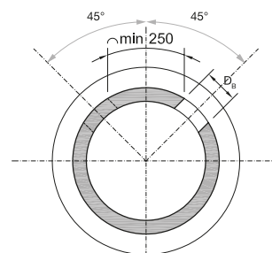
D_B = Diametru gaură de foraj
