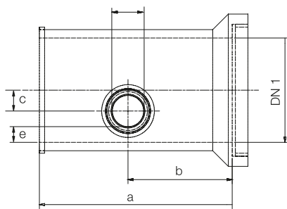
Ramificație fără mufă 90° grade
