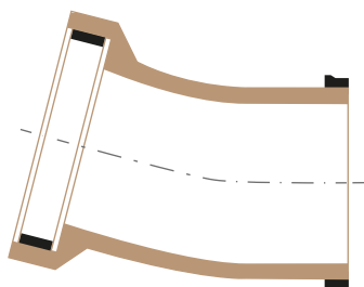
Cot 15° cu mufă de conectare K
