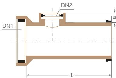
Ramificație compactă 90°
