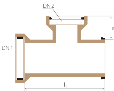
Ramificație 90°
