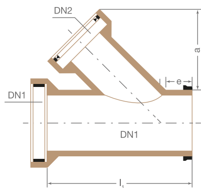
Ramificație 45°
