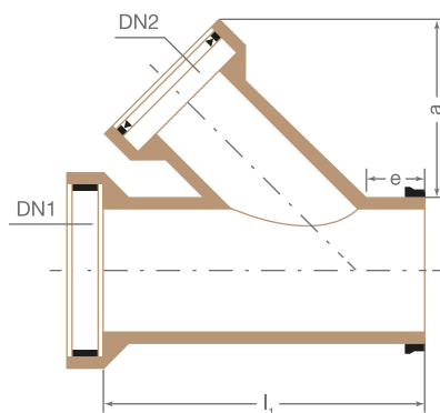
Ramificație 45°
