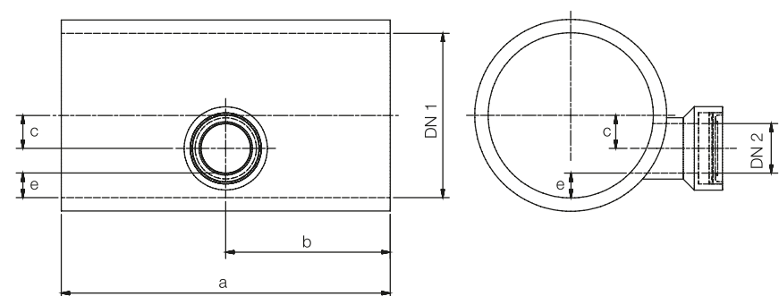
Ramificație excentrică: conductă principală fără mufă/admisie cu mufă
