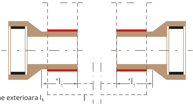
Montare piesă articulată (GE)
