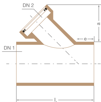
Ramificație reparație 45°
