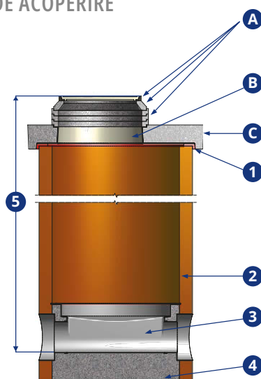
CĂMIN DE VIZITARE DN 800 PANĂ LA DN 1000 CU PLACĂ DE ACOPERIRE
