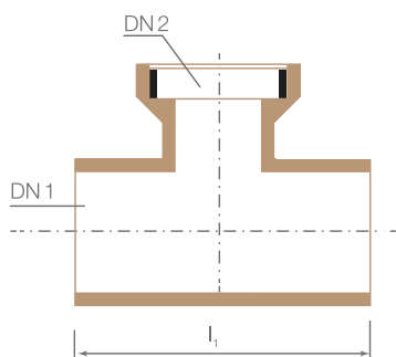
Ramificație specială 90° DN 1 fără mufă, DN 2 cu mufă
