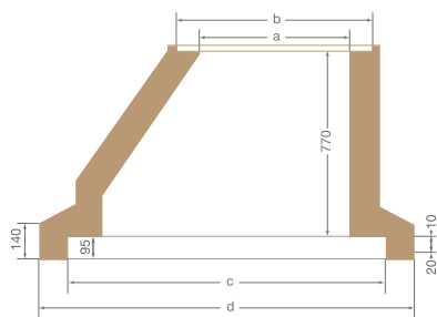
KERA.Port Konus für Schächte DN 1000
