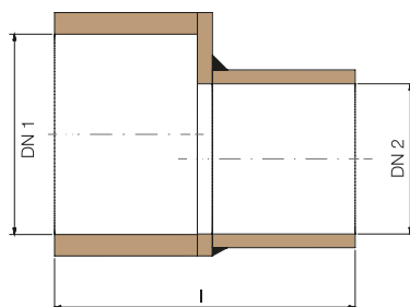
Secțiune longitudinală
