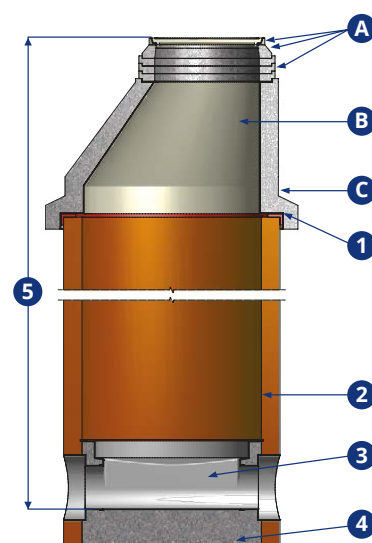
CĂMIN DE VIZITARE DN 1000 CU CON
